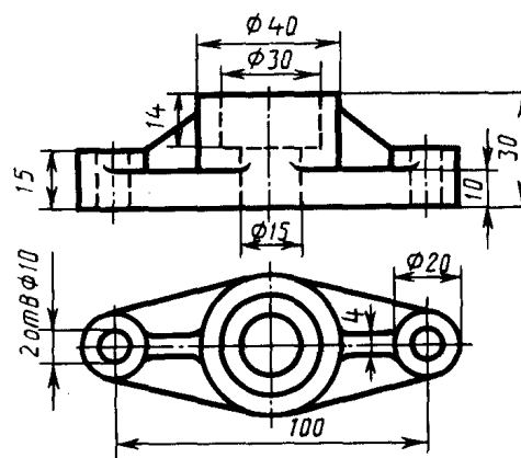
Фланец
