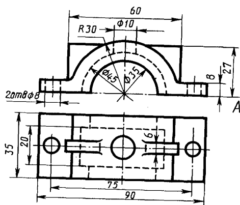
Крышка
