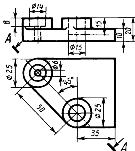
Плита
