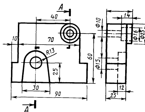
Стойка
