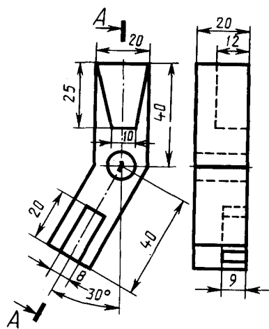
Угольник
