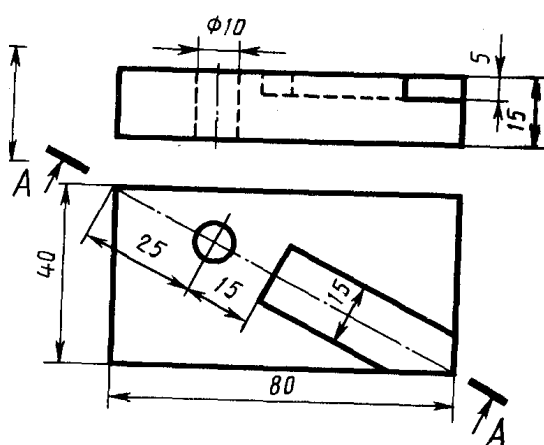
Плита
