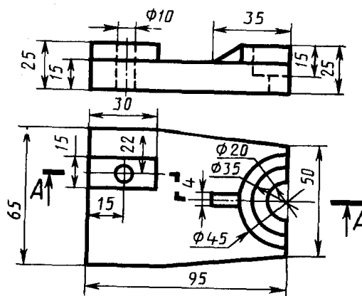
Опора
