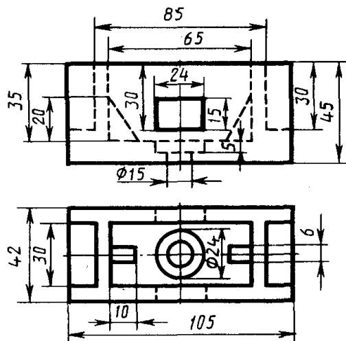
Коробка
