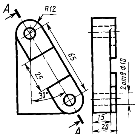
Пластина
