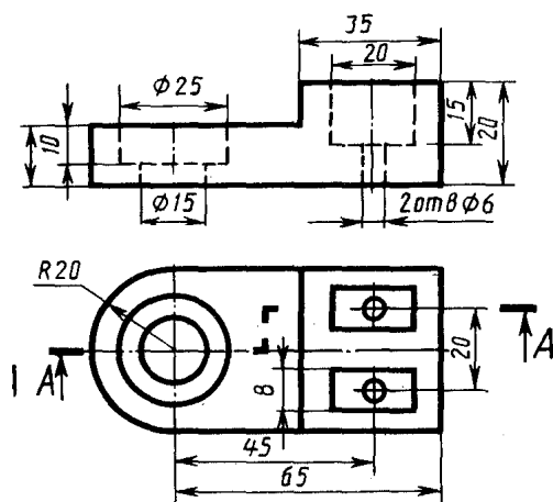
Упор
