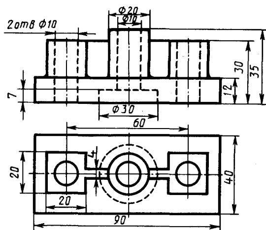
Опора
