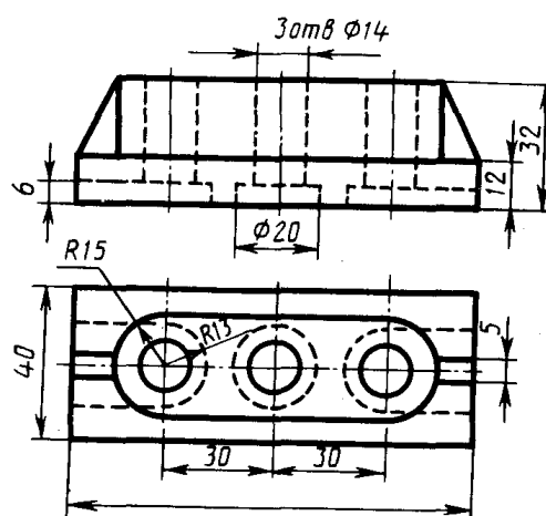
Опора
