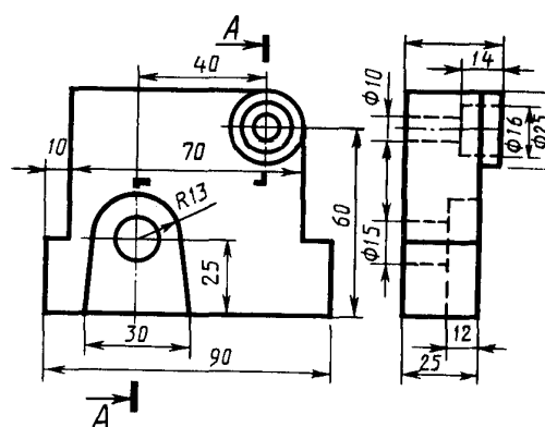
Стойка
