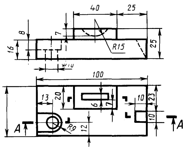
Брус
